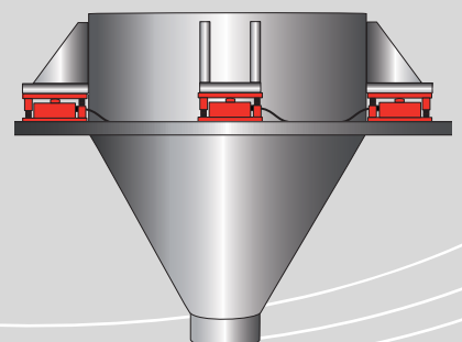
CP压式传感器和安装模块KCPN
