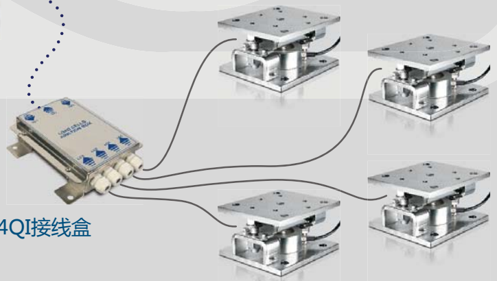
CP压式传感器和安装模块KCPN
